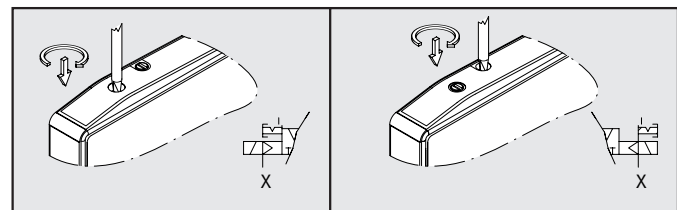
BIESTABLE MANUAL CONECTOR 2 con actuación directa sobre la bobina
