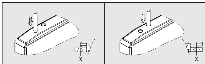
MONOESTABLE MANUAL CONECTOR 2 con actuación directa sobre la bobina
