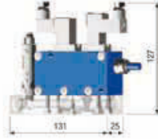
[1] Generatore di vuoto Vacuum generator GVMM 10/14
